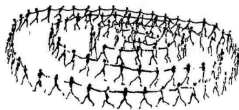
Universele cirkelbeweging
